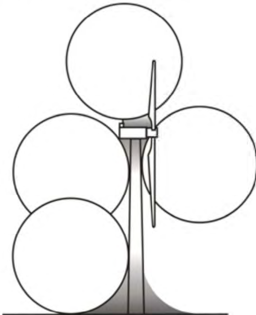
Abbildung 3.1: Das „Rollkugelverfahren“
