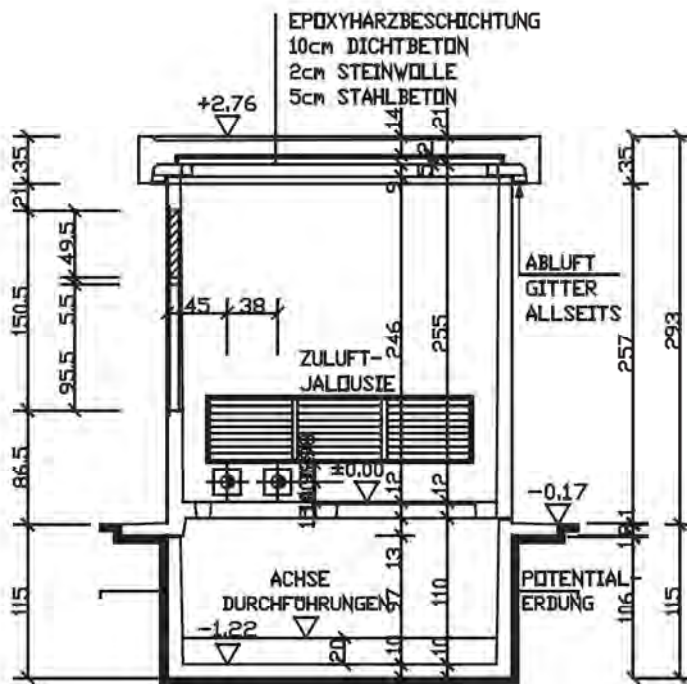
SCHNITT C-C
