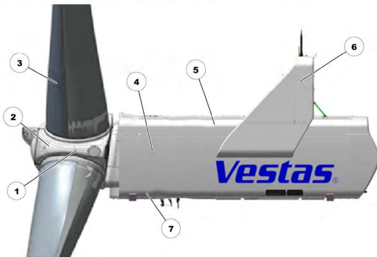
Abbildung 7.2: Maschinenhausbereiche
