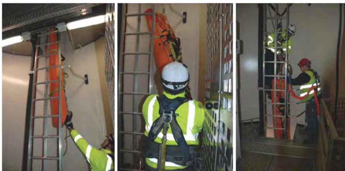
Abbildung 7.23: Die Person beim Absenken führen, wenn die Abstiegsvorrichtung verwendet wird
