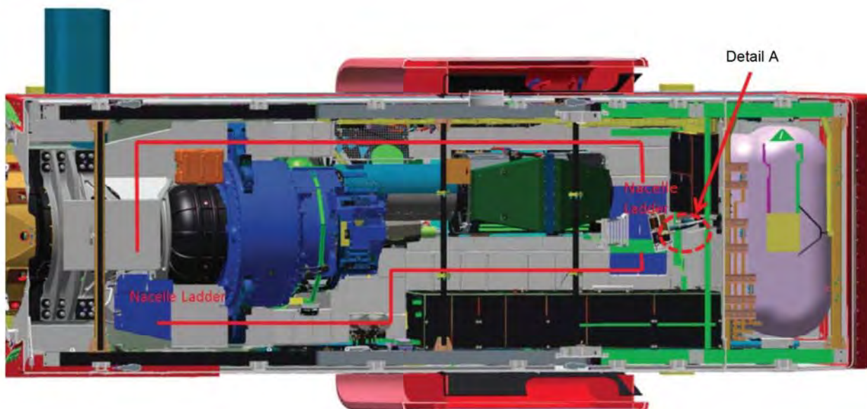
Abbildung 7.17: Rettungsroute im Maschinenhaus
