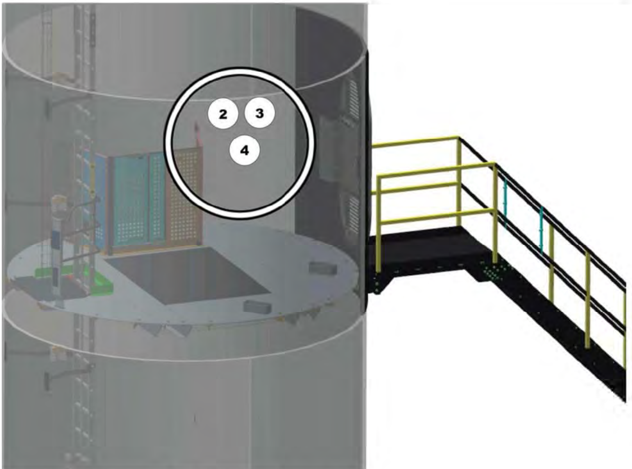
Abbildung 8.2: Standort der Sicherheitsausrüstung im Turm
