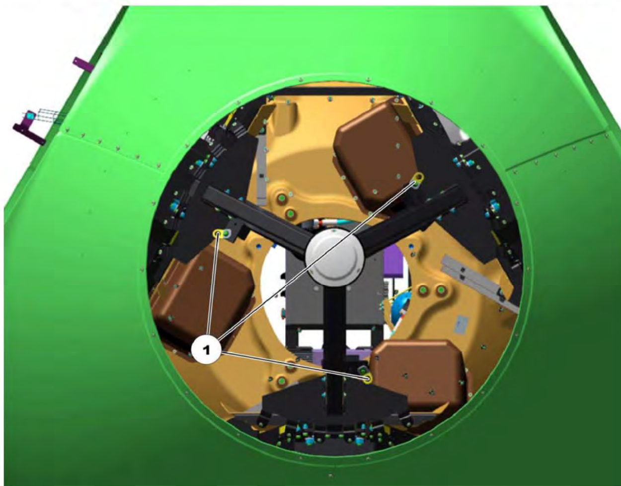
Abbildung 7.14: Verankerungspunkte nahe der Luken in der Nabenabdeckung
