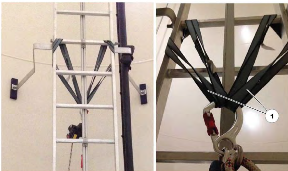
Abbildung 7.21: Die Abstiegsvorrichtung mit 2 Schlingen an der Leiter befestigen
