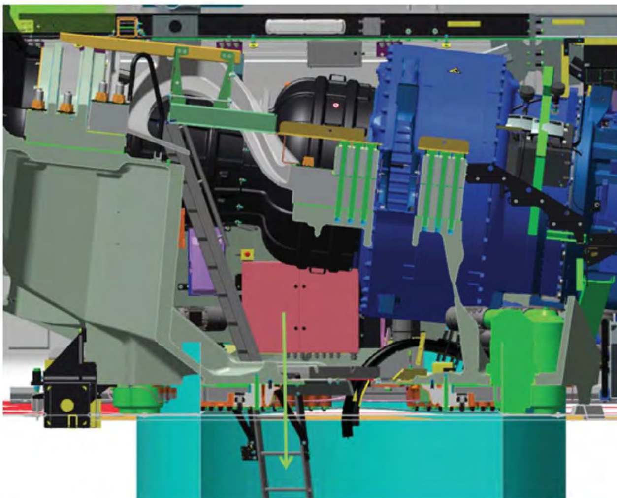
Abbildung 7.11: Evakuierungsrouten vom Yawdeck
