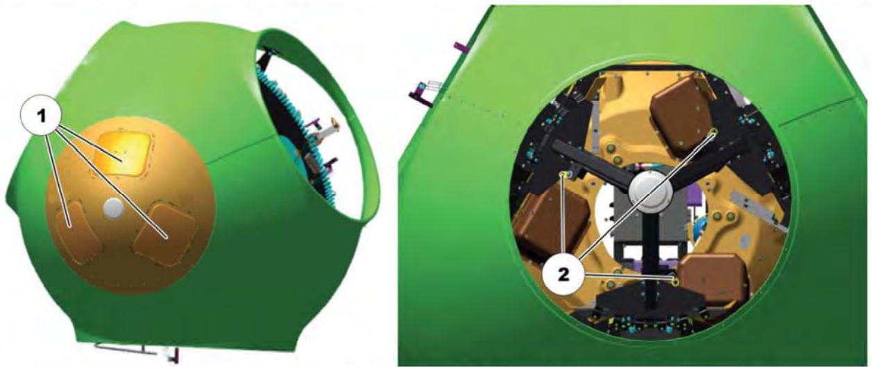
Abbildung 7.16: Rettungsroute durch die Spinnerluken und Verankerungspunkte für Abstiegsvorrichtung
