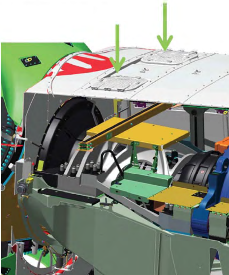
Abbildung 7.10: Vorderseite, Dachlukenzugang
