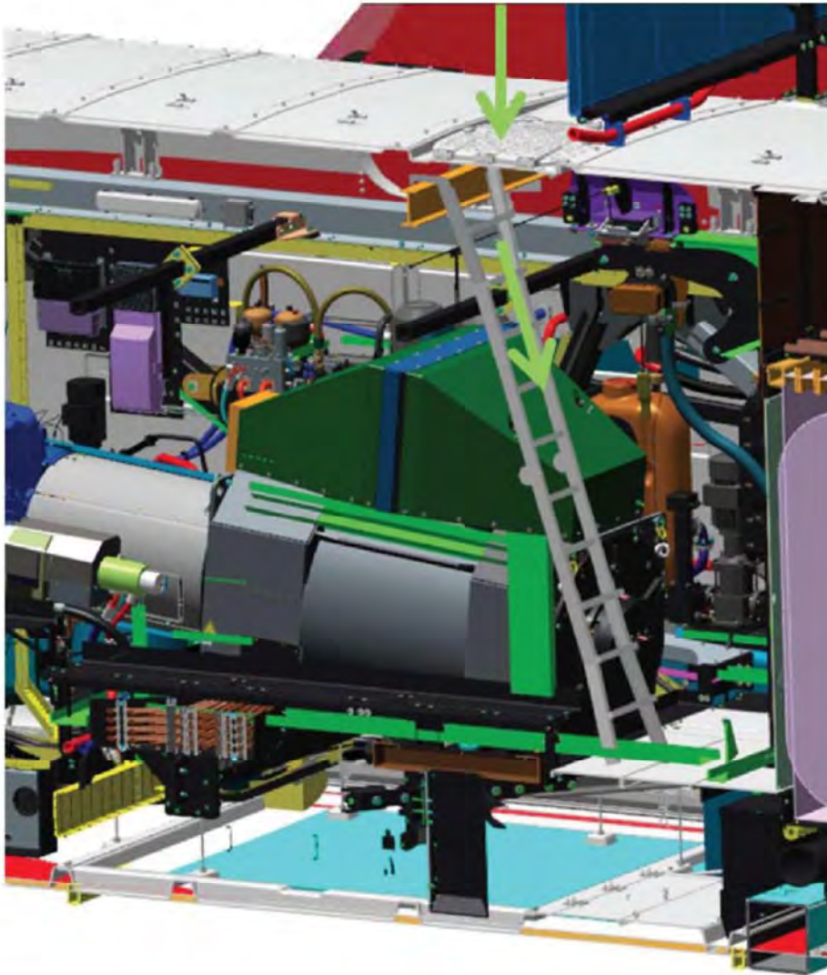
Abbildung 7.9: Hinteres Ende, Dachlukenzugang
