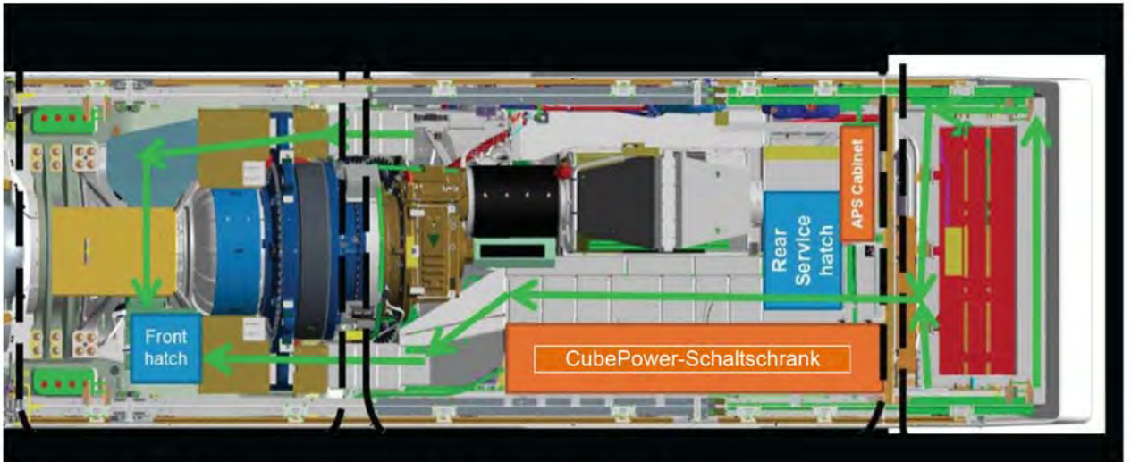
Abbildung 7.6: Evakuierungsrouten im Maschinenhaus
