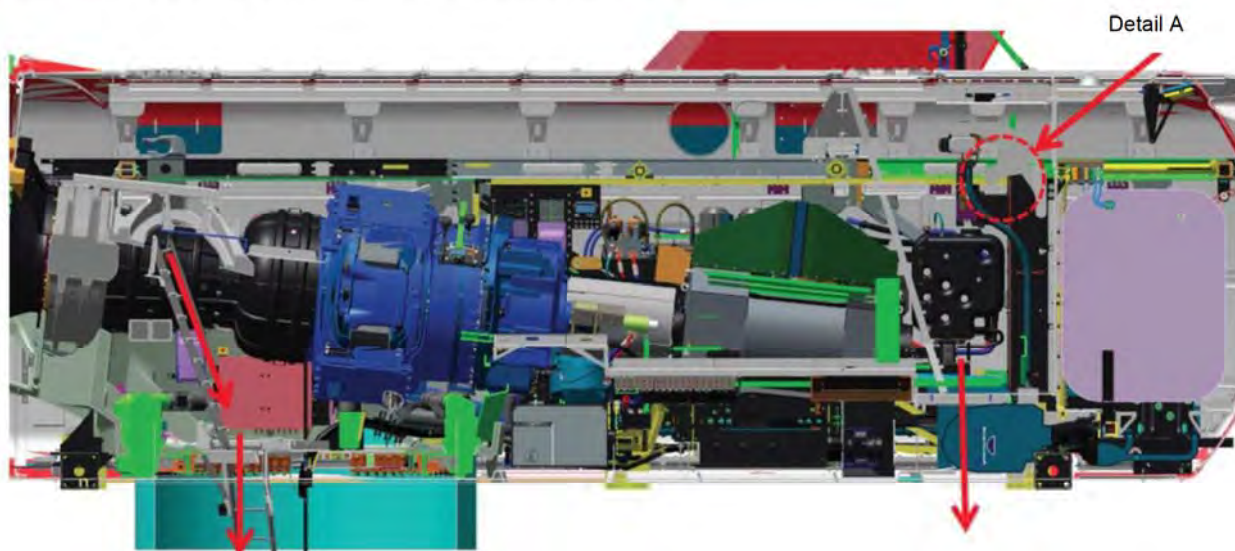
Abbildung 7.18: Rettungsroute im Maschinenhaus
