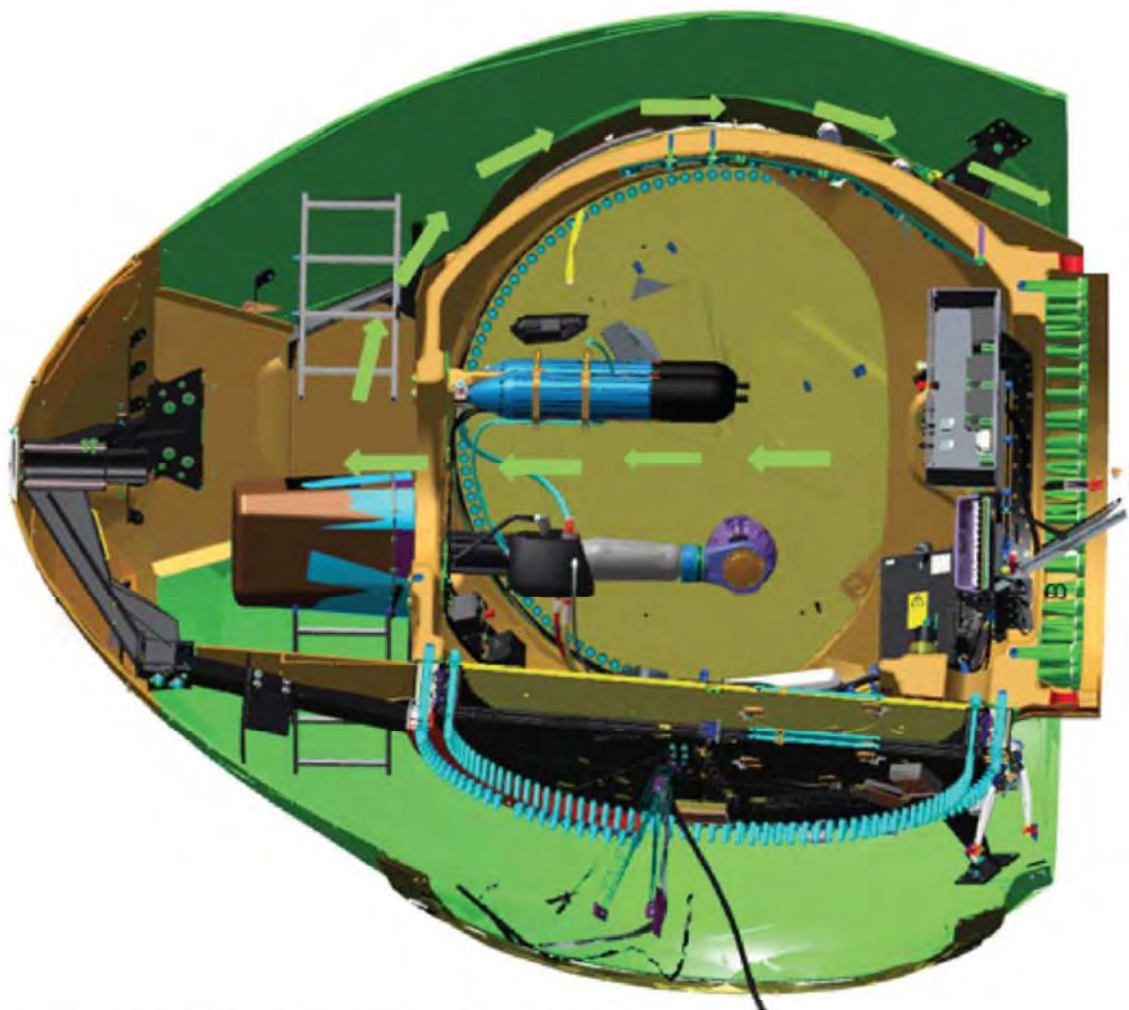
Abbildung 7.5: Evakuierungsroute in der Nabe
