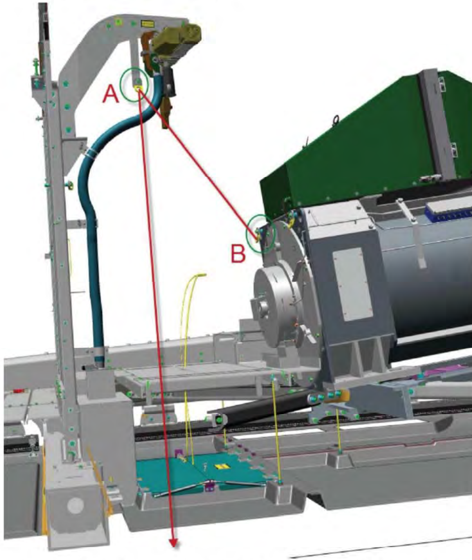
Abbildung 7.19: Rettungsroute im Maschinenhaus (Detailansicht)
