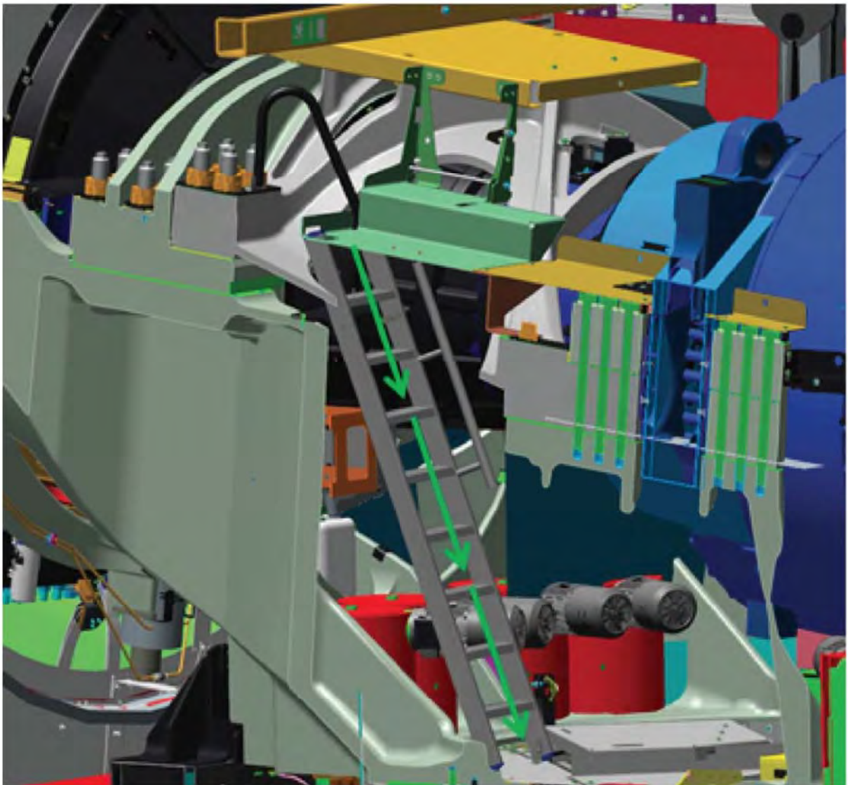
Abbildung 7.7: Leiter zum Yawdeck
