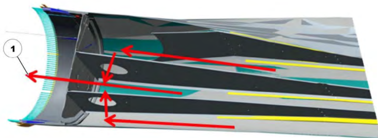
Abbildung 7.15: Rettungsrouten innerhalb des Rotorblatts (Rotorblatt in horizontaler Position arretiert)
