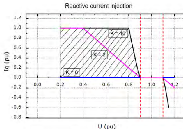
Abbildung 10-6: Blindstromeinspeisung
