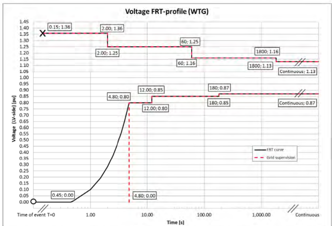
Abbildung 10-5: Spannungstoleranzkurve für symmetrische und asymmetrische Störungen, wobei U die gemessene Spannung im Stromnetz darstellt.
