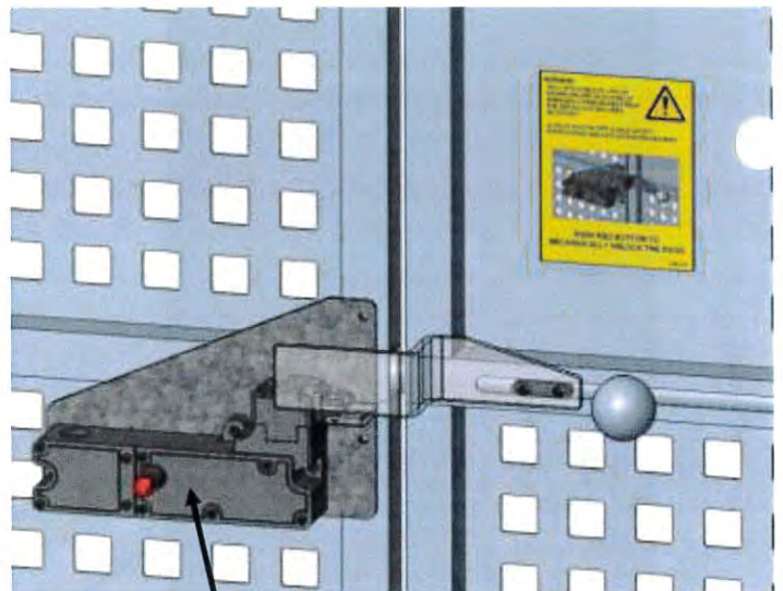
Türwächter
