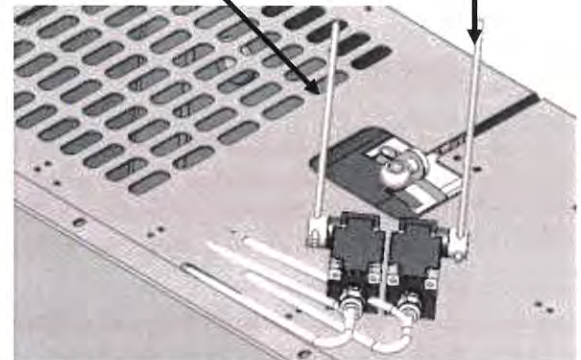
Not-Endschalter
