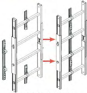
Flanschverbindingssatz
