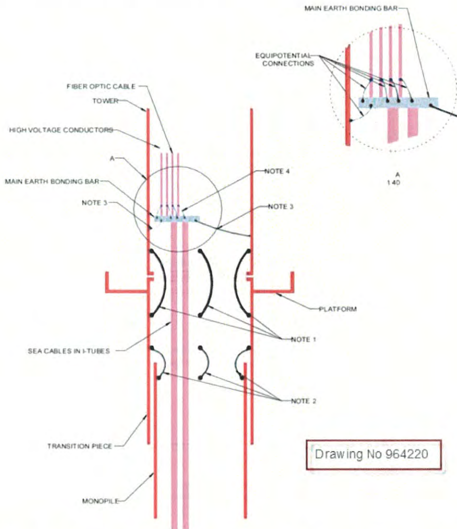
Abbildung 3.13: Prinzipdarstellung des Vestas-Erdungssystems bei I-Rohr-Aufstellung
