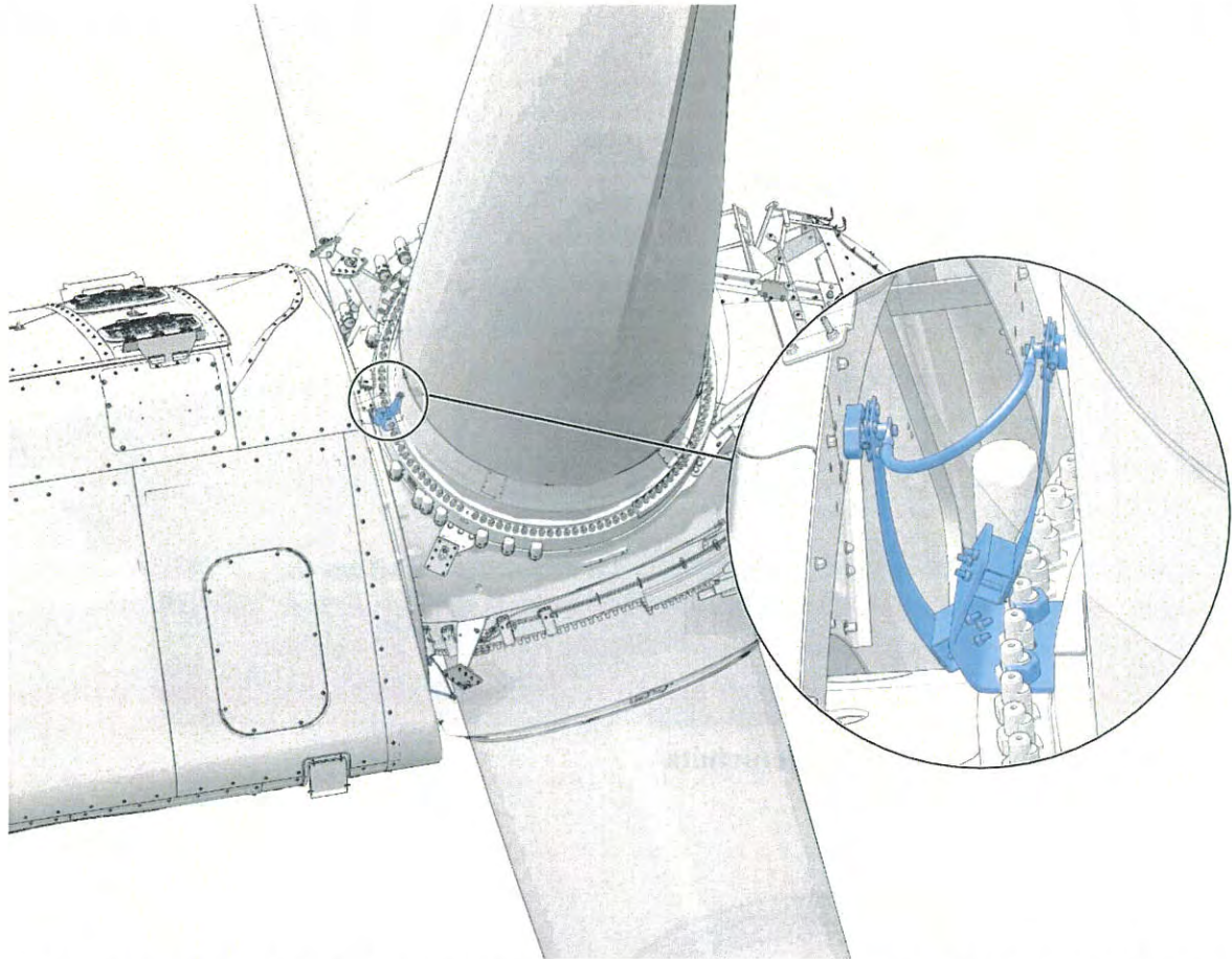
Abbildung 3.6: Blitzstromableiter zwischen den Rotorblättern und der Maschinenhausstruktur
