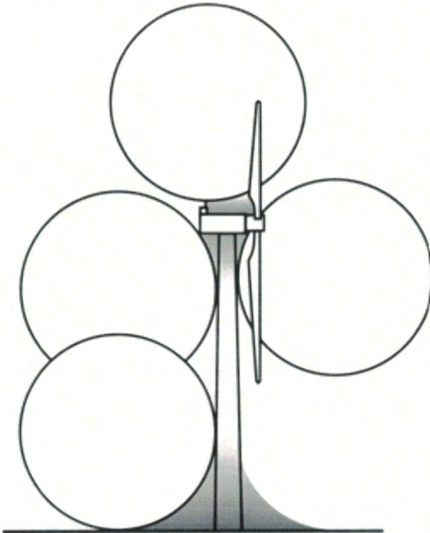
Abbildung 3.1: Das „Rollkugelverfahren“
