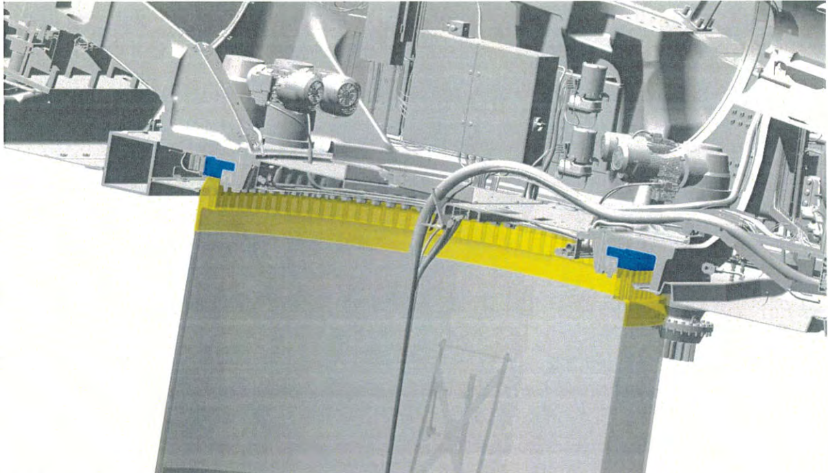
Abbildung 3.7: Azimutlagerschutz
