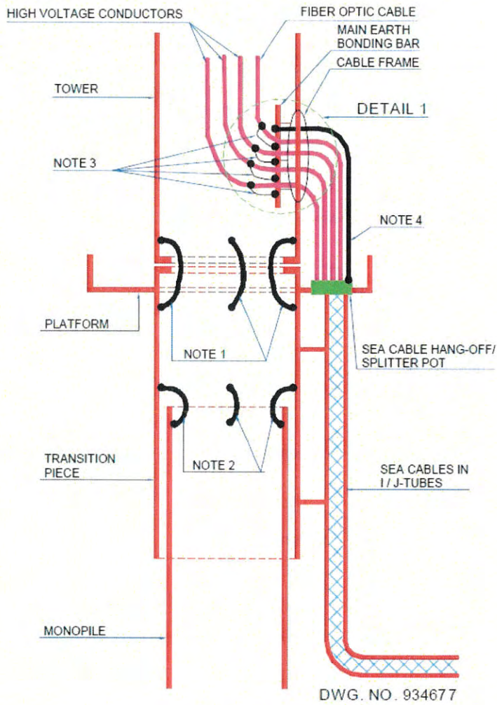
Abbildung 3.12: Prinzipdarstellung des Vestas-Erdungssystems bei J-Rohr-Aufstellung
