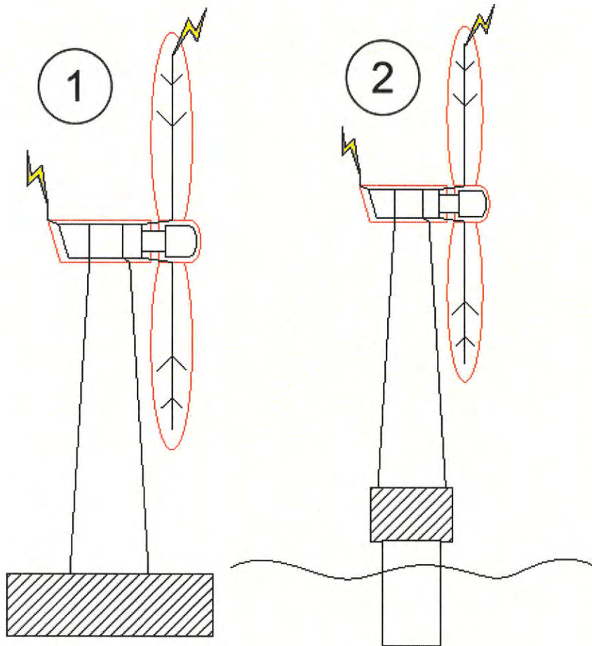
Abbildung 3.2: Blitzschlagpunkte und Blitzableitungssystem
