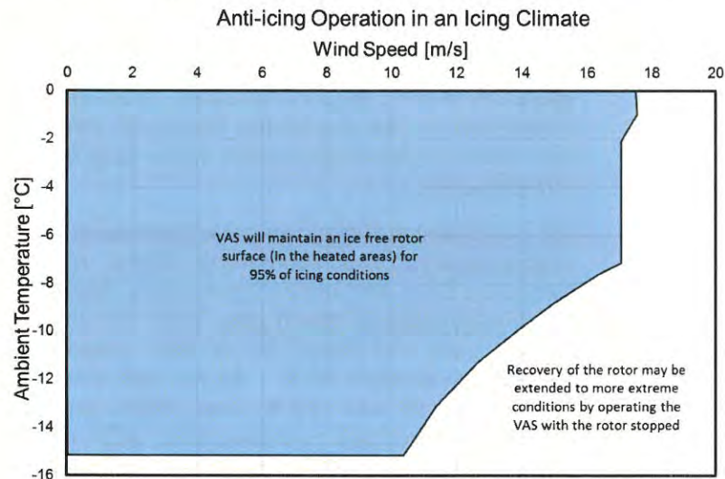
Abbildung 5. Klimatische Abhängigkeit der VAS-Leistungsgrenze für 95 % aller Vereisungsbedingungen an einem Standort mit starkem Eisverlust in nordischen Ländern.
