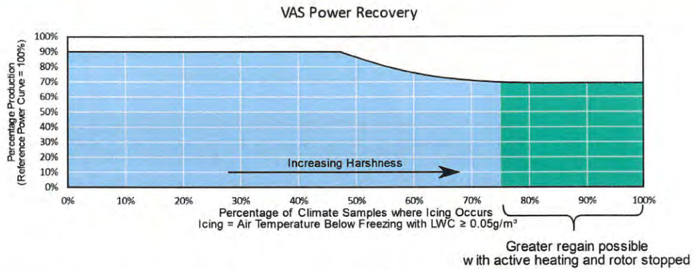
Abbildung 6. VAS-Stromrückgewinnung in Prozent aller Vereisungsstunden an einer repräsentativen schweren Vereisungsstelle (> 8 % Vereisungsverlust bei der jährlichen Energieproduktion).
