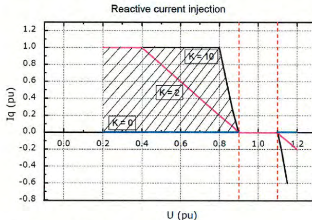
Abbildung 10-6: Blindstromeinspeisung
