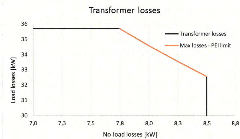
Abbildung 4-1 Transformatorverluste – zulässiger Bereich
