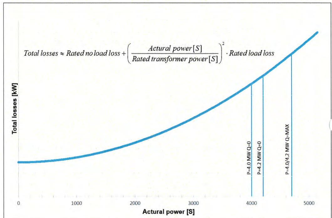
Abbildung 4-2: Gesamtverluste gegenüber tatsächlicher Leistung.
