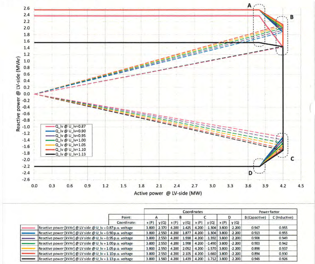
Abbildung 10-4: Die Blindleistungskapazität im leistungsoptimierten 4,2-MW-Modus (PO1).
