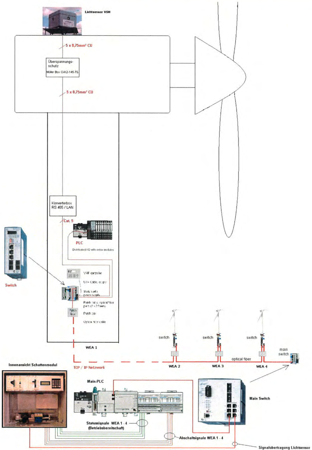
Abbildung 12-1: Prinzipskizze „Einbindung in die VestasOnline™ Fernüberwachung“
