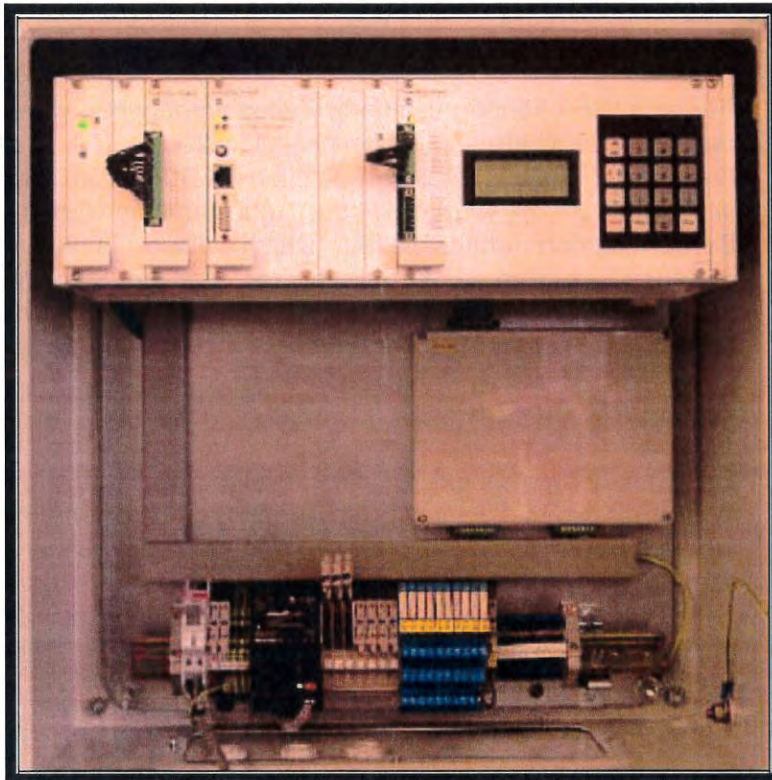
Abbildung 10-2: Schattenwurfmodul Innenansicht
