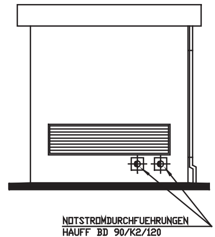
SEITENANSICHT
