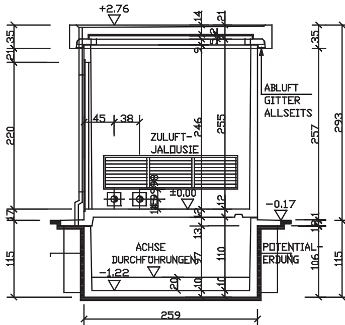
SCHNITT B-B
