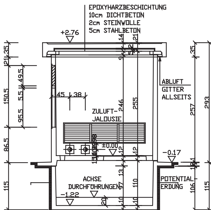
SCHNITT C-C
