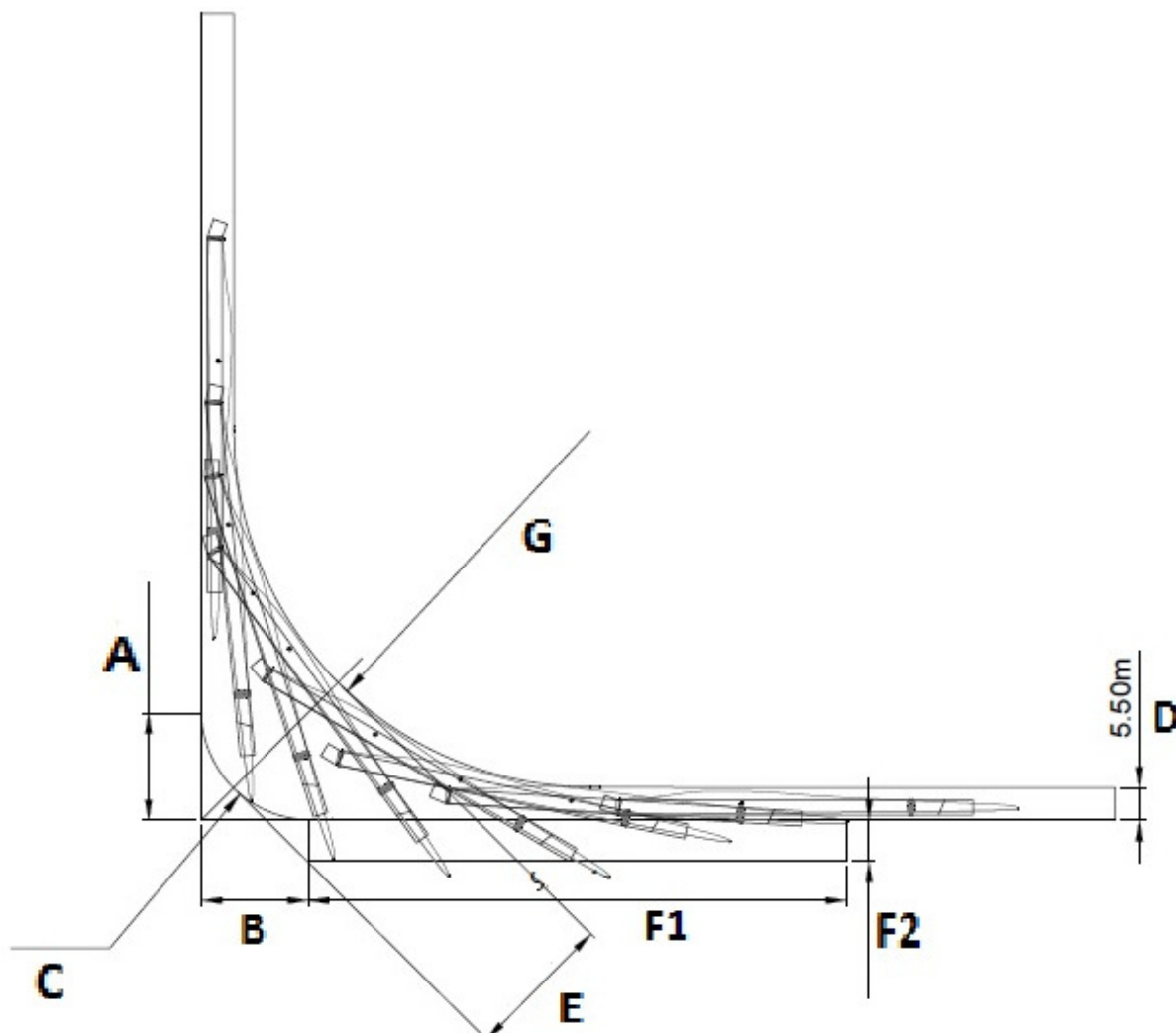
Abbildung 8: Darstellung einer 90°-Kurve
