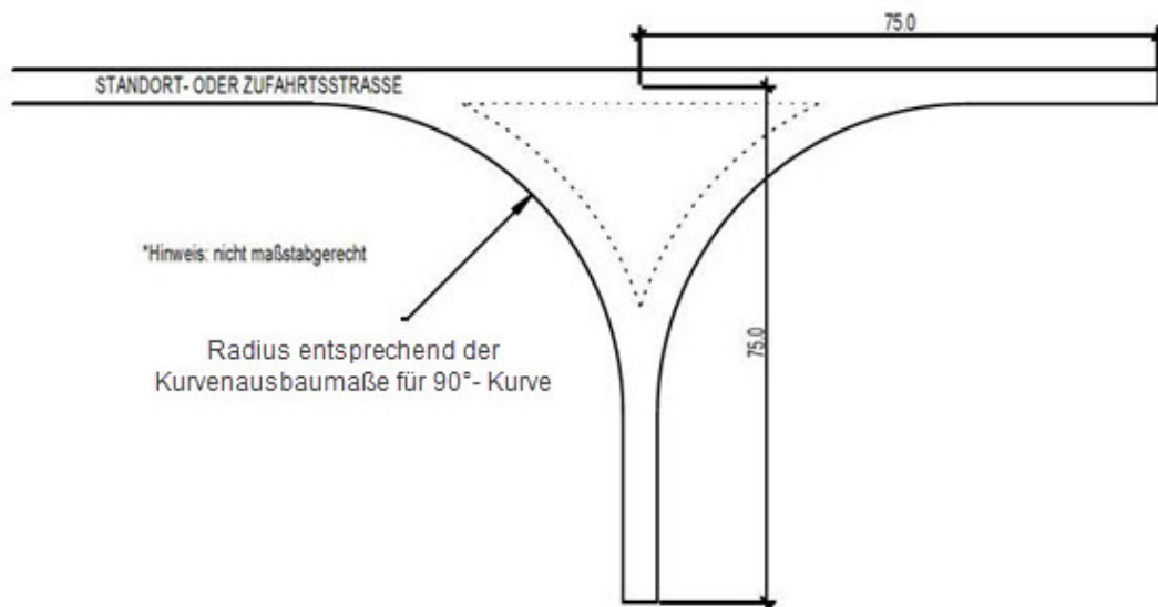
Abbildung 11: Wendemöglichkeit mit einer Rückfahrlänge von \geq 75 m
